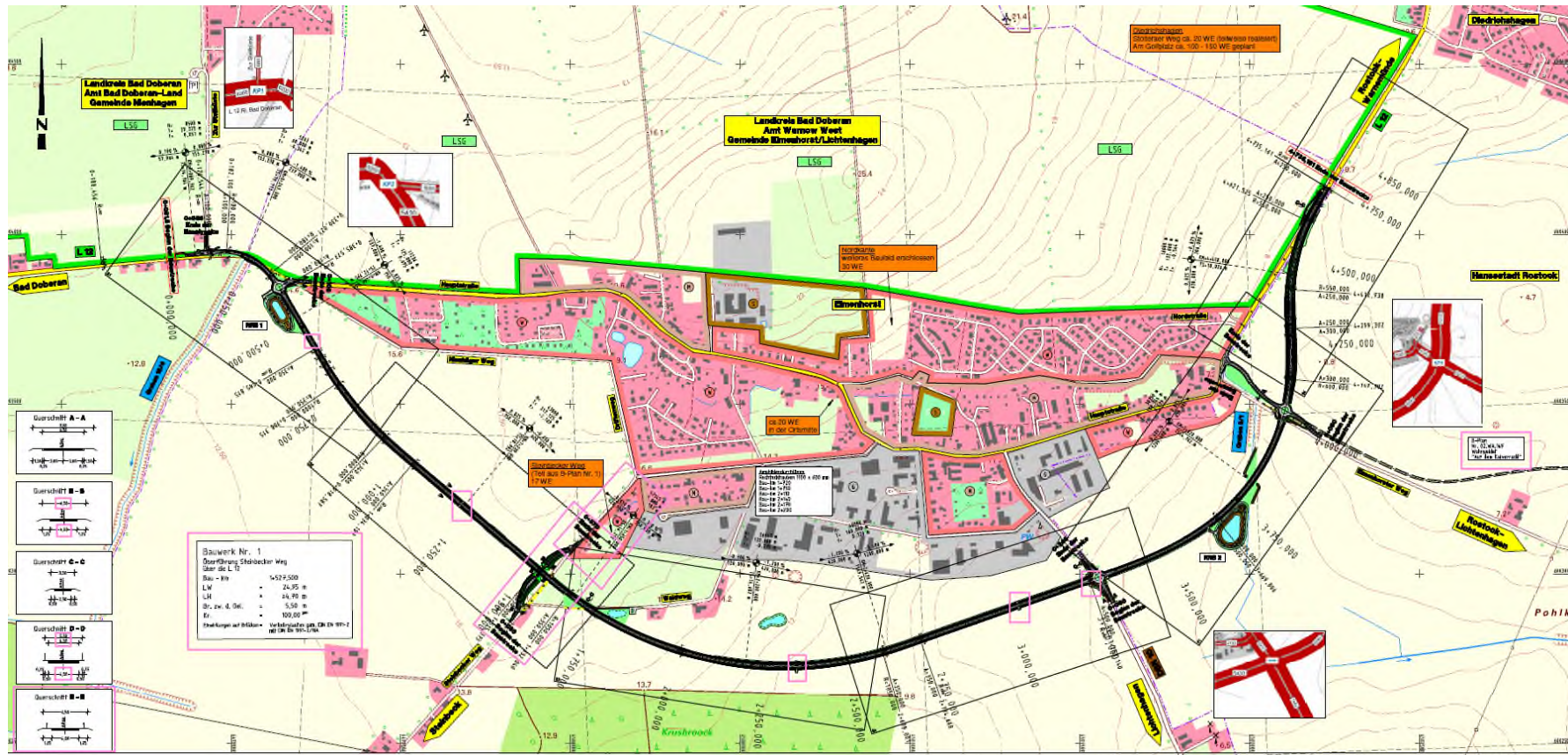
Auszug Planungsunterlage
